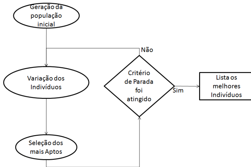
Figura 1.3: Algoritmo Evolutivo Básico
