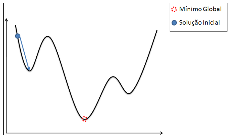
Figura 1.2: Busca Local numa Função Multimodal
