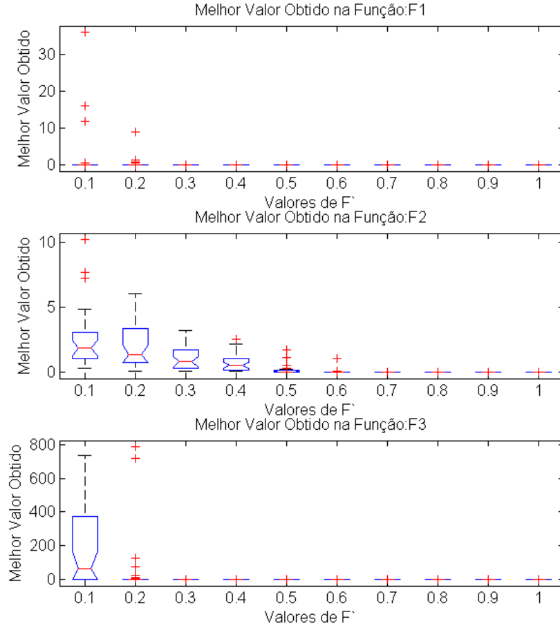
Figura 4.2: Melhor Valor Encontrado em Média nas Funções Unimodais Variando F'
