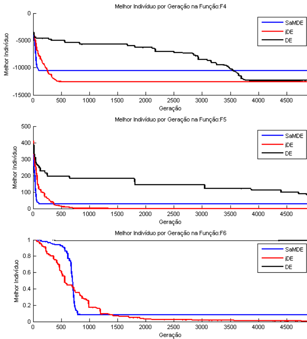
Figura 4.17: Comportamento do Melhor Indivíduo da População nas Funções Multimodais
