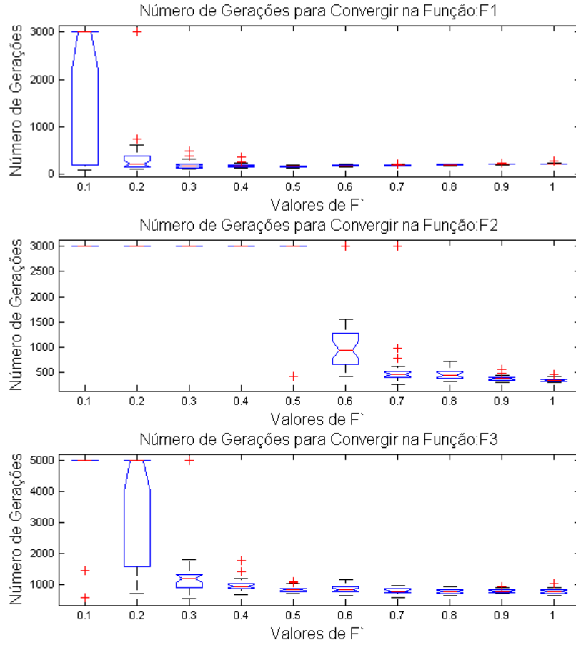
Figura 4.1: Número de Gerações Gastos em Média para Convergência nas Funções Unimodais Variando F'
