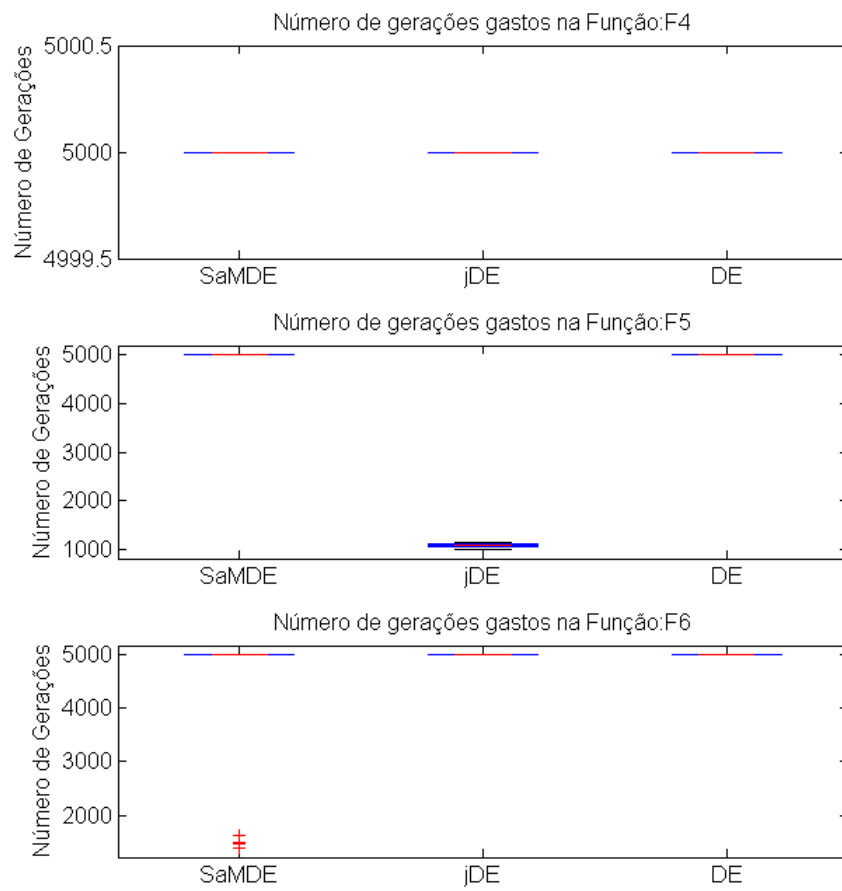
Figura 4.14: Número de Gerações gastas em Média nas Funções Multimodais
