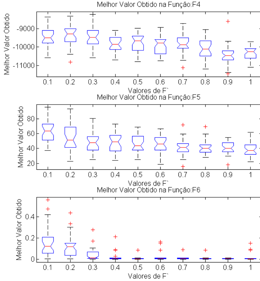
Figura 4.3: Melhor Valor Encontrado em Média nas Funções Multimodais Variando F'
