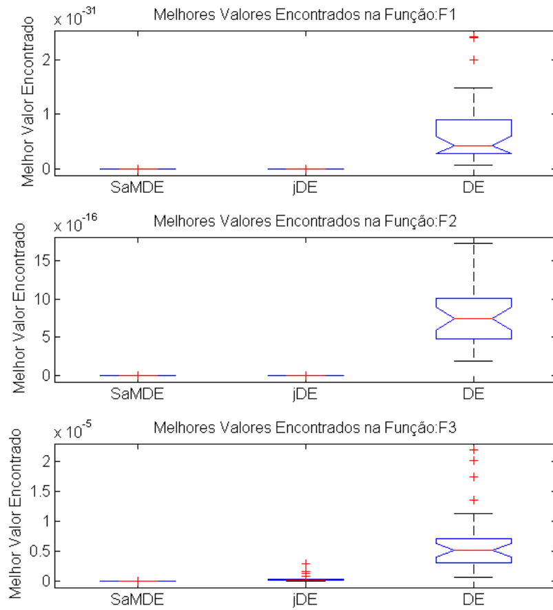
Figura 4.13: Melhor Valor Encontrado em Média nas Funções Unimodais
