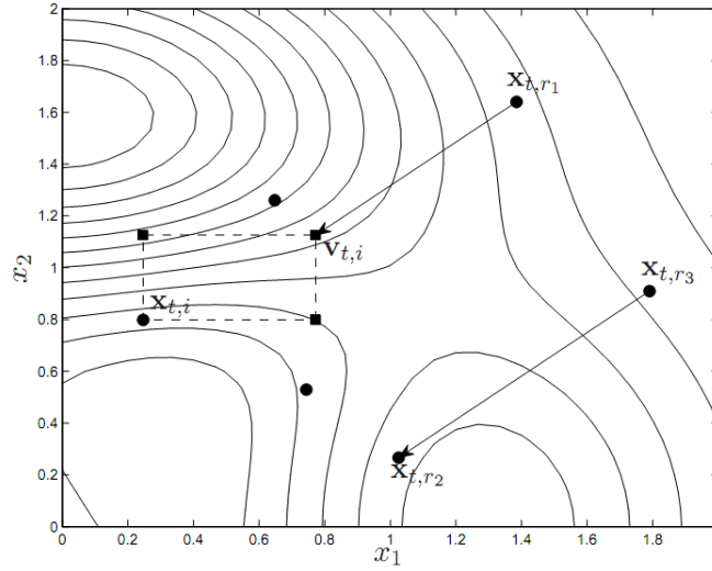
Figura 2.1: Ilustração do procedimento de geração de uma solução mutante (Guimarães, 2009)
