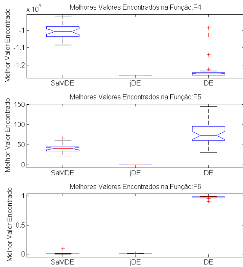
Figura 4.15: Melhor Valor Encontrado em Média nas Funções Multimodais
