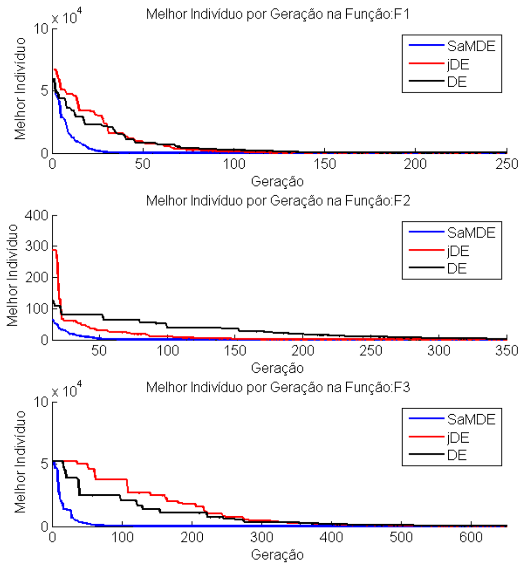
Figura 4.16: Comportamento do Melhor Indivíduo da População nas Funções Unimodais
